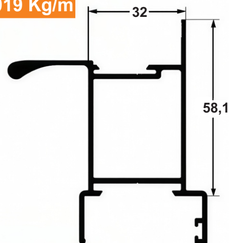
LG 020 1,019 Kg/m
