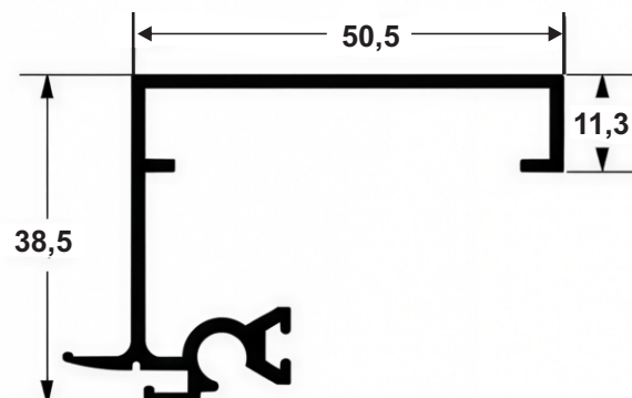
FA 258 0,592 Kg/m
