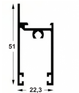
SU 053 0,469 Kg/m
