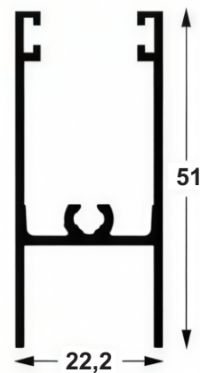
SU 187 0,492 Kg/m
