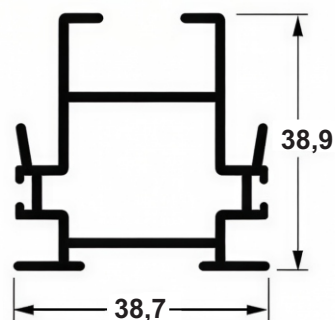
SU 057 0,638 Kg/m
