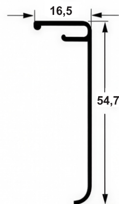
BX 108 0,244 Kg/m
