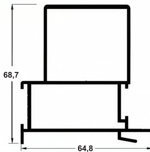
SU 289 1,359 Kg/m
