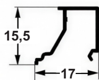
ME 024 0,568 Kg/m
